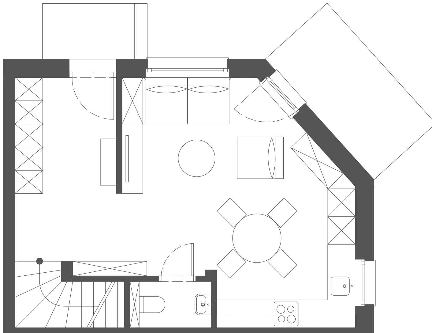
parter 35,25 m 2 | SUCHY LAS | UL. ZIELIŃSKIEGO | lokal B | dz. nr 106/35 | skala: 1-50
