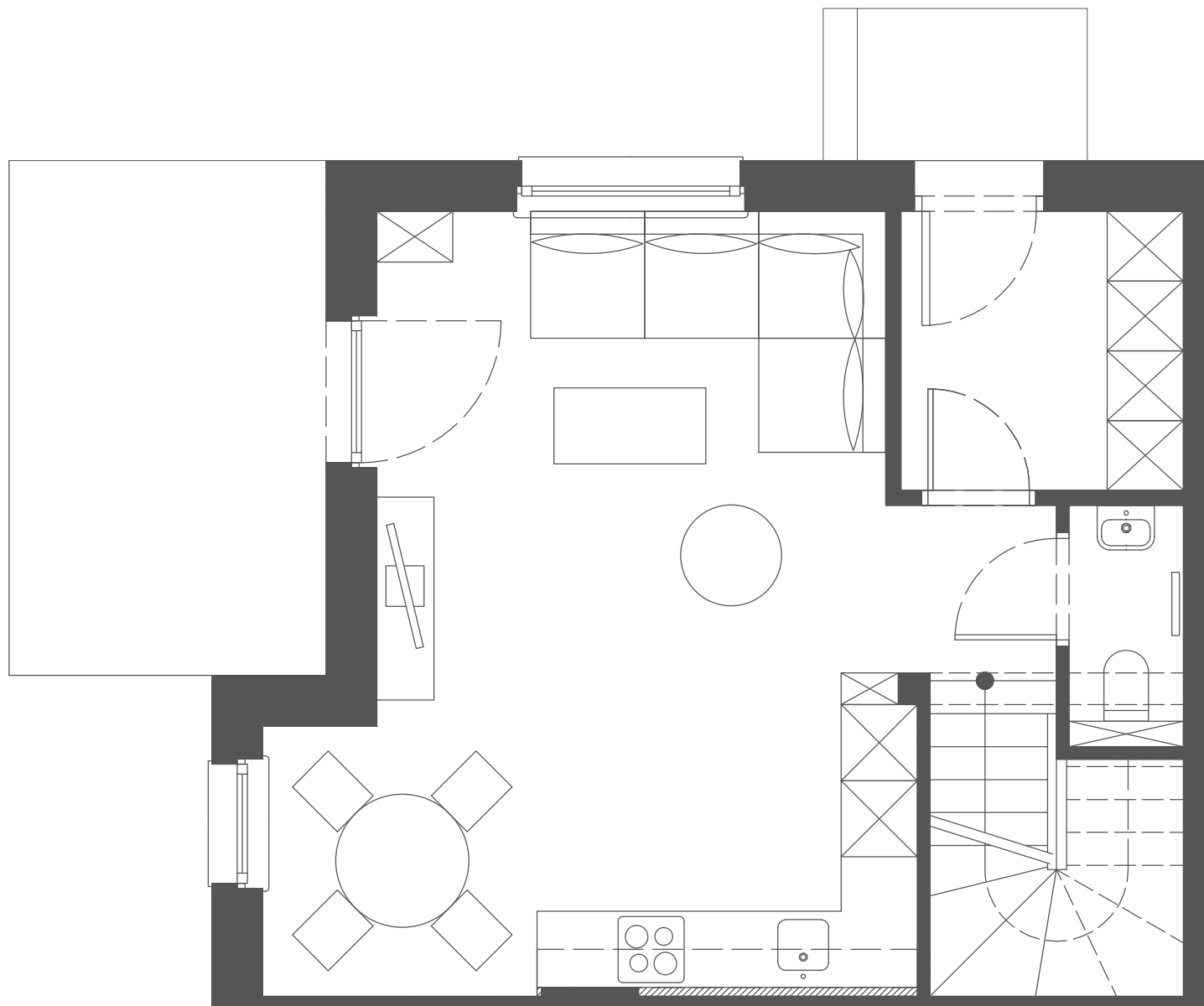
parter 38,62 m2 | SUCHY LAS | UL. ZIELIŃSKIEGO | lokal B | dz. nr 106/36 | skala: 1-50
