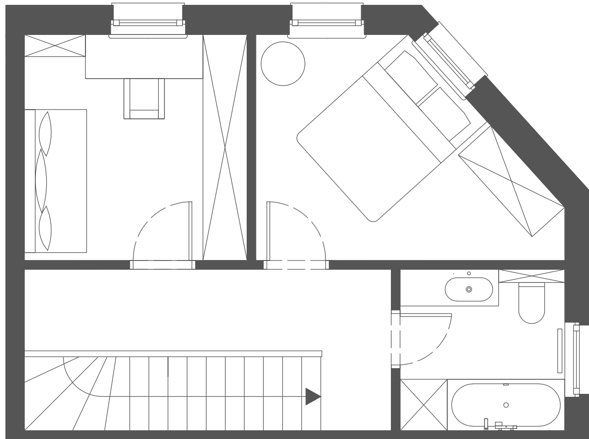
piętro 35,22 m 2 | SUCHY LAS | UL. ZIELIŃSKIEGO | lokal B | dz. nr 106/35 | skala: 1-50
