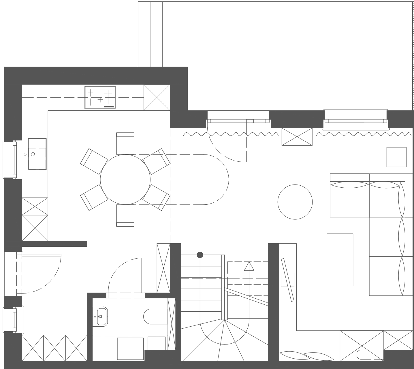
parter 49,22 m 2 | SUCHY LAS | UL. ZIELIŃSKIEGO | lokal B | dz. nr 106/37 | skala: 1-50
