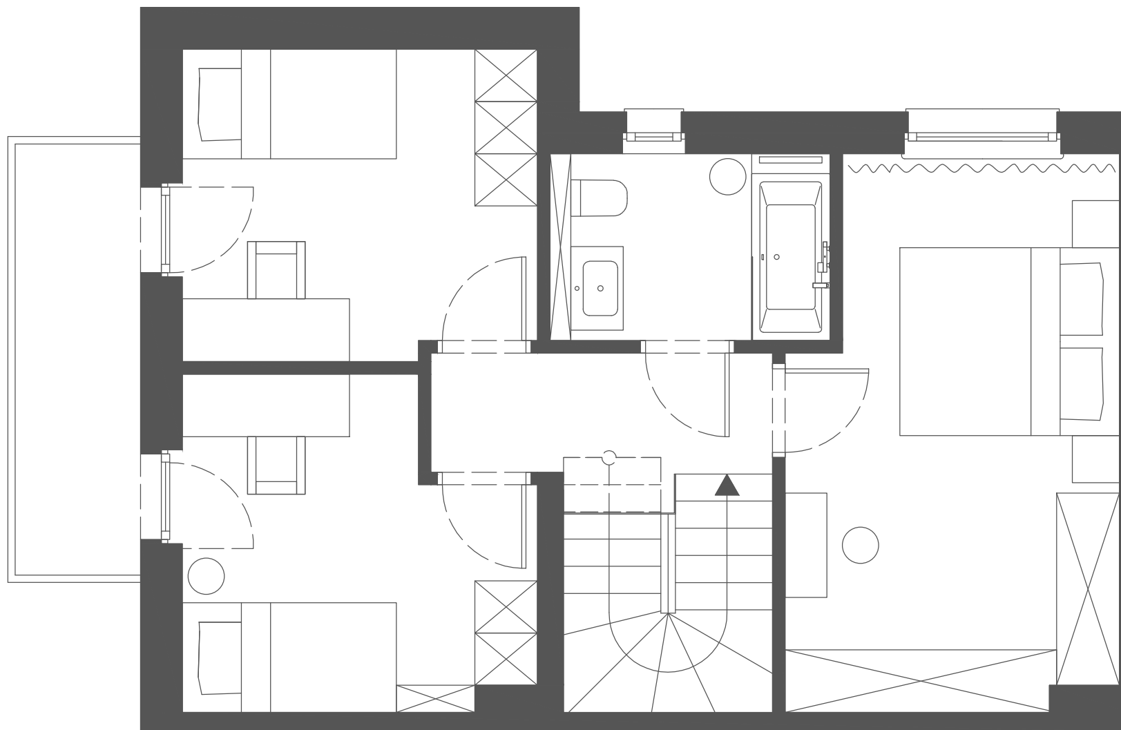
piętro 48,55 m 2 | SUCHY LAS | UL. ZIELIŃSKIEGO | lokal B | dz. nr 106/37 | skala: 1-50
